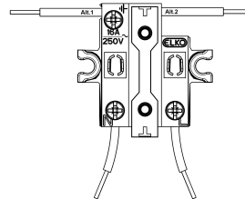
Koblingskjema
