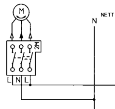
Koblingskjema
