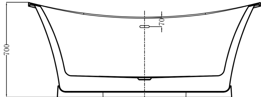
SECTION D-D
