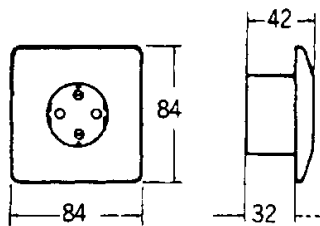
Målskisse
