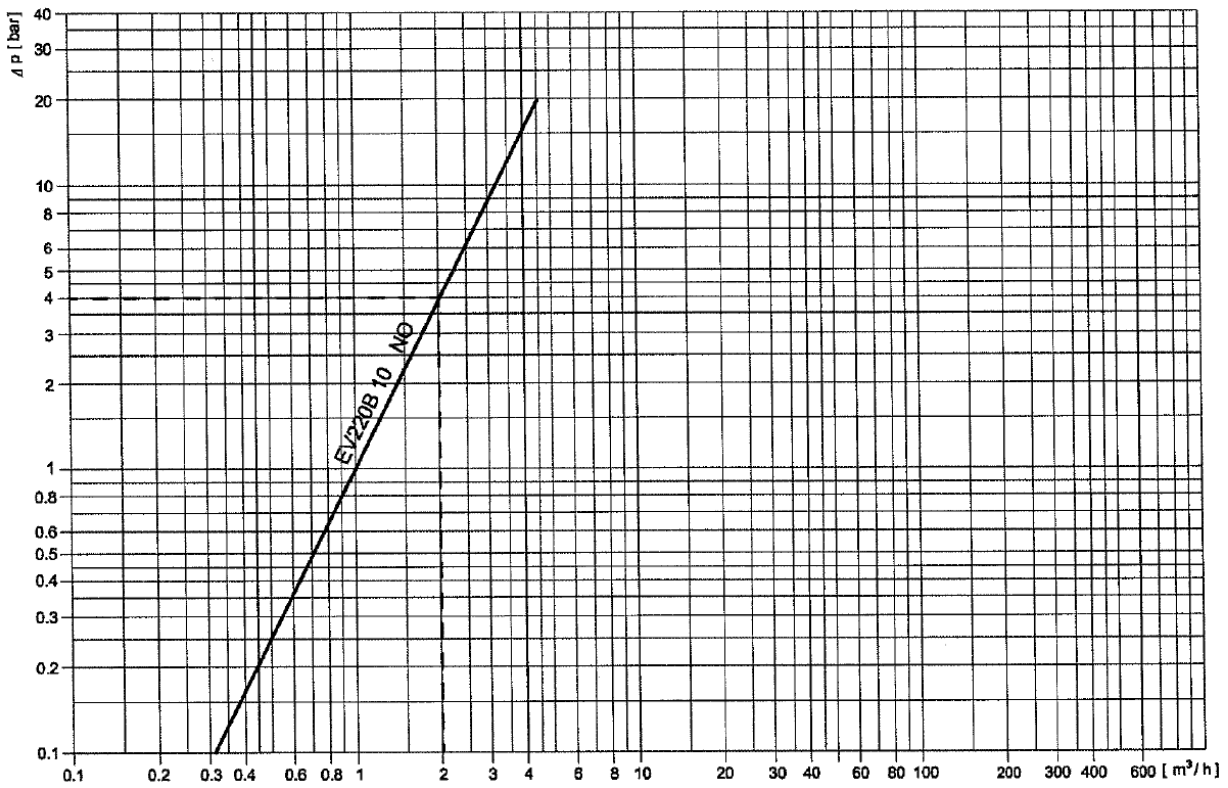
Trykkfallsdiagram 1/2'' ventil:
