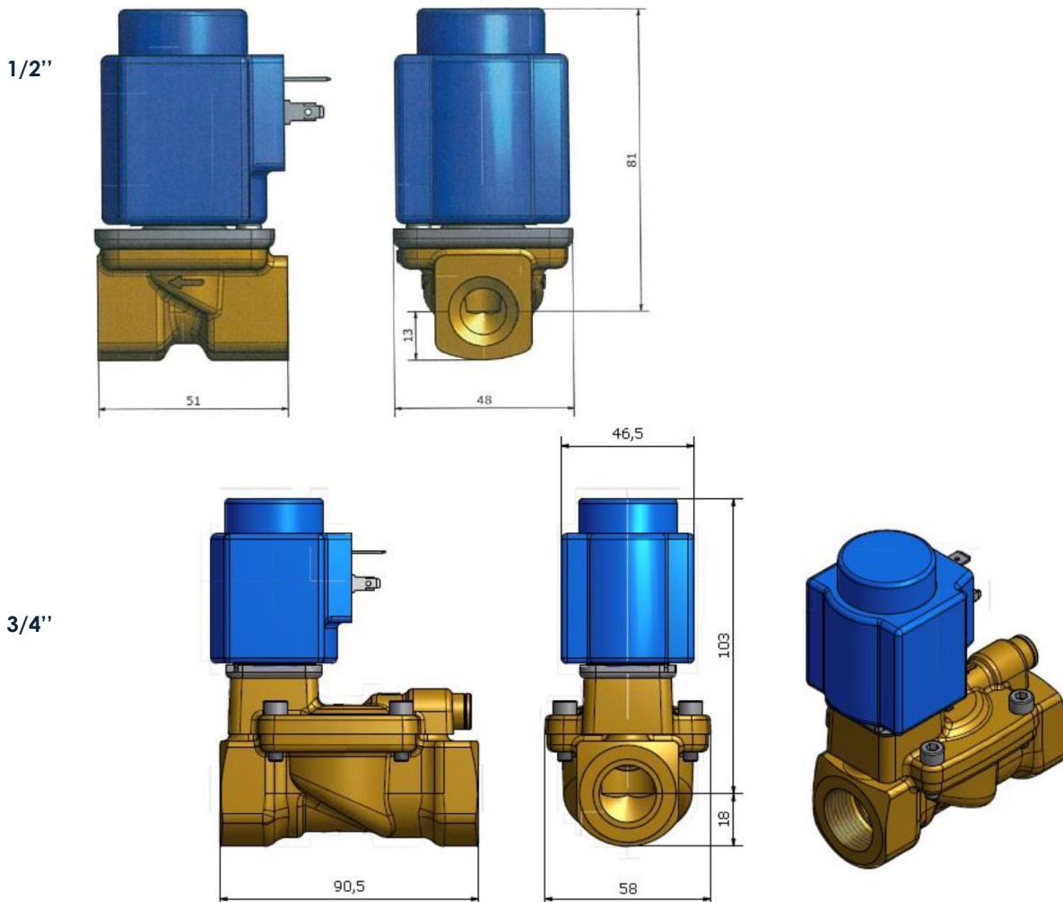
Målskisser ventil med coil:
