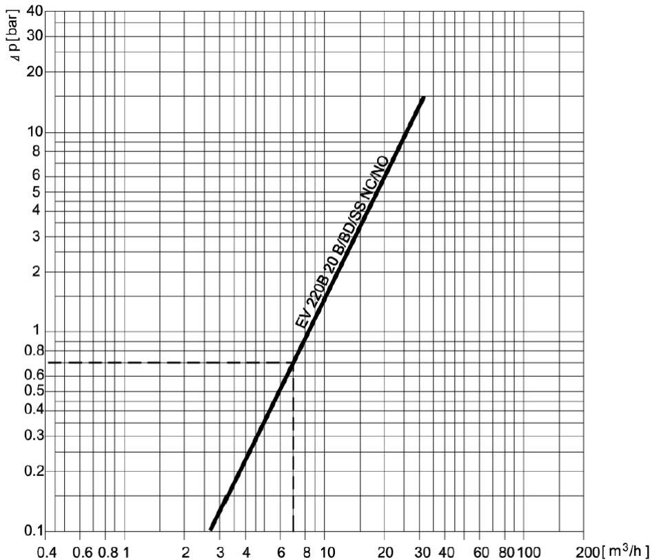
Trykkfallsdiagram 3/4'' ventil:
